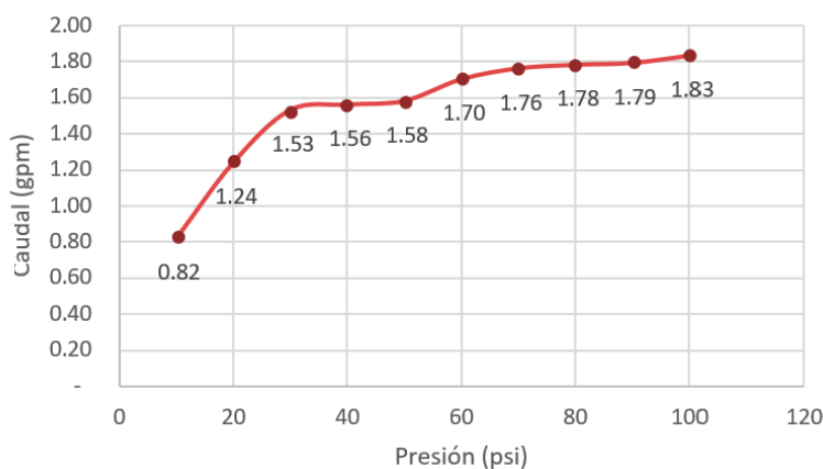
Gráfica de flujo
